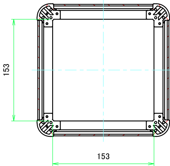
C-C ( 1:3.5 )
